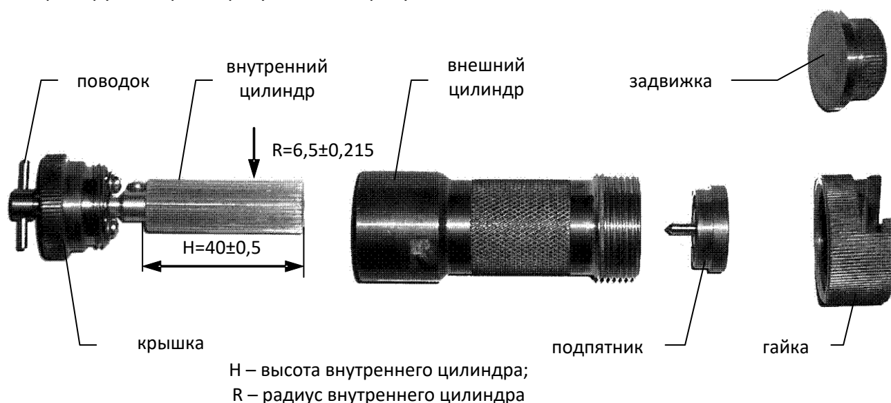
Рисунок 1 – Элементы датчика
